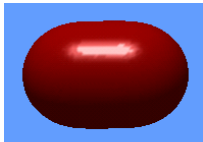
\sigma_{1s}
