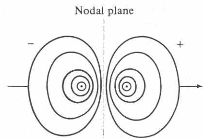
\sigma^*_{1s}
