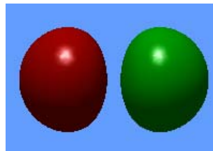
\sigma^*_{1s}
